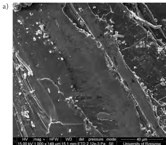
Ryc. 8. Wyniki analizy składu chemicznego (EDS) rdzenia siekierki w obszarze 2; a) mikrostruktura, b) spektrogram
