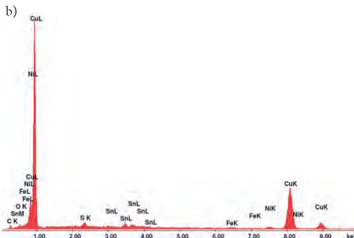
Ryc. 9. Wyniki analizy składu chemicznego (EDS) rdzenia siekierki w obszarze 3; a) mikrostruktura, b) spektrogram
