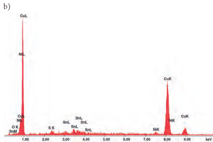
Ryc. 8. Wyniki analizy składu chemicznego (EDS) rdzenia siekierki w obszarze 2; a) mikrostruktura, b) spektrogram
