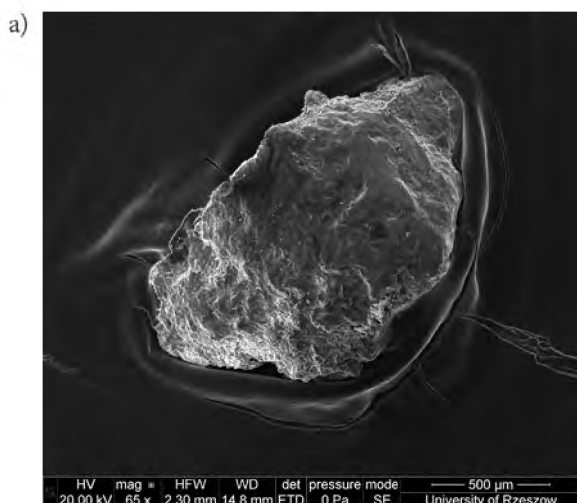
Ryc. 10. Wyniki analizy składu chemicznego (EDS) warstwy wierzchniej siekierki; a) mikrostruktura, b) spektrogram
