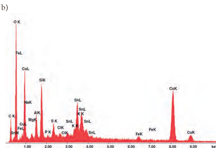
Ryc. 10. Wyniki analizy składu chemicznego (EDS) warstwy wierzchniej siekierki; a) mikrostruktura, b) spektrogram
