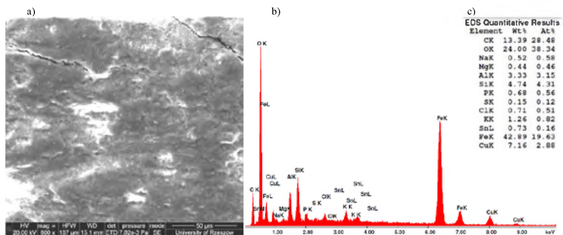
Ryc. 8. Analiza składu chemicznego (EDS) warstwy wierzchniej siekierki: a) mikrostruktura, b) widmo sygnału EDS, c) stężenie pierwiastków – pomiar 3. Opr. A. Dziedzic
