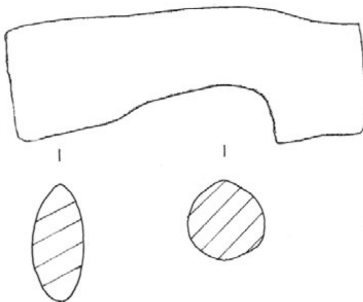
Tabl. XVIII. Przemyśl, Pl. Katedralny, stan. 20. Kamienna forma odlewnicza po złożeniu dwóch części oraz rekonstrukcja siekiery wraz z przekrojami
