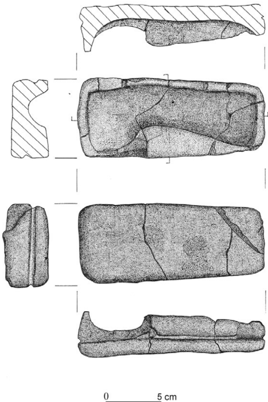
Tabl. XVII. Przemyśl, Pl. Katedralny, stan. 20. Kamienna forma odlewnicza z warstwy osadniczej – część górna Table XVII. Przemyśl, Cathedral Sq., site No. 20. Stone casting mould from the settlement layer – the upper part
