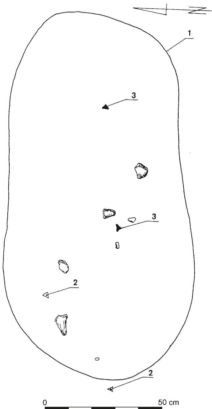
Ryc. 343. Wojciechowice, pow. Opatów. Stanowisko I. Plan obiektu 58.
