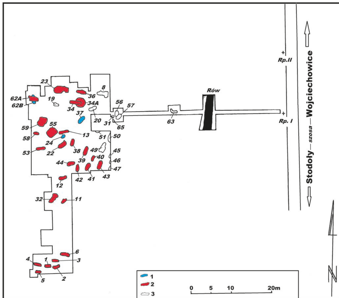
Ryc. 266b. Wojciechowice, pow. Opatów. Stanowisko I, wykop IV. Plan cmentarzyska KCS, Ch-V i KM. 1 – groby KCS, 2 – przebadane groby Ch-V i KM, 3 – groby nieprzebadane. Grafika Jerzy T. Bąbel.
