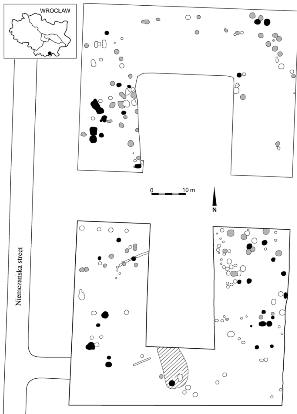
Fig. 8. Wrocław-Niemczańska street; general plan of the settlement with chronology of the features marked gray (the older phase) and black (the younger phase). Ryc. 8. Wrocław, ul. Niemczańska; plan ogólny osady z zaznaczonymi fazami chronologicznymi obiektów. Kolor szary (faza starsza), kolor czarny (faza młodsza).
