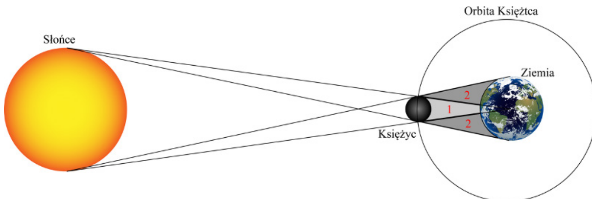
Rys.1. Schemat geometryczny obrazujący zaćmienie Słońca. Na rysunku przyjęto następujące oznaczenia:
