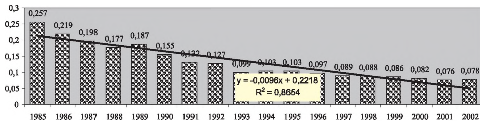
Rysunek 4. Wartości odchylenia standardowego logarytmów ilorazów syntetycznych mierników poziomu życia ludności dla każdego z czternastu krajów UE i średniej dla Unii w latach 1985–2002 oraz oszacowana na jego podstawie funkcja trendu liniowego.
